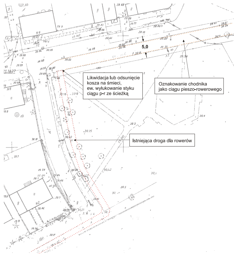
Rysunek 14 Przebieg drogi dla rowerów przez skwer u zbiegu ulic Wojciechowskiego i Traktorzystów Skala 1 : 1 000
