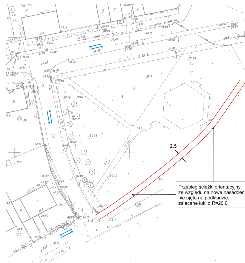
Rysunek 14 Przebieg drogi dla rowerów przez skwer u zbiegu ulic Wojciechowskiego i Traktorzystów Skala 1 : 1 000
